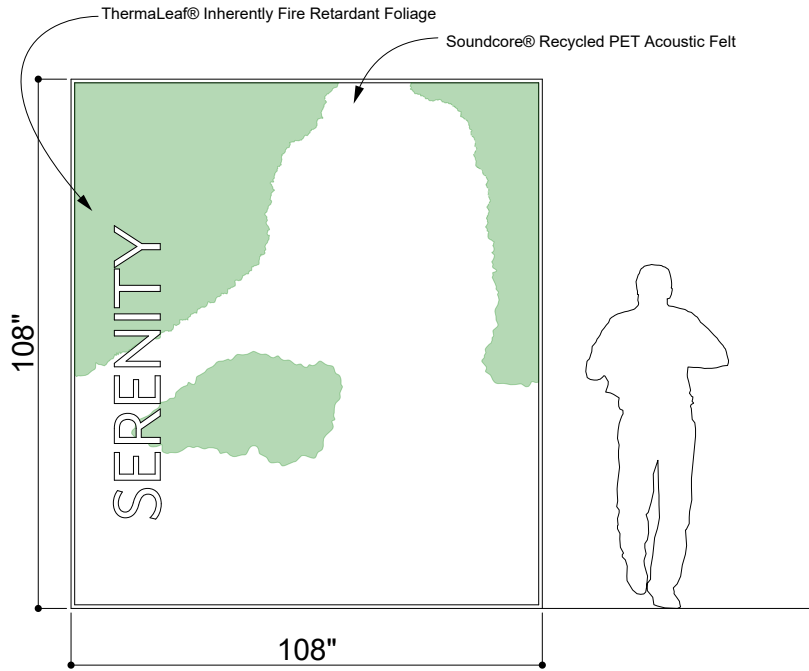
① ELEVATION 1
